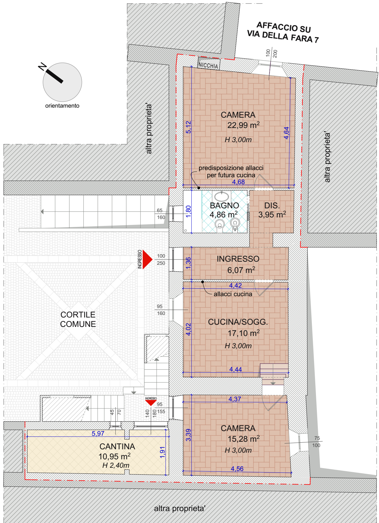
PIANO PRIMO - Scala 1:100
