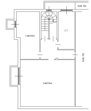
PIANO PRIMO SOTTOSTRADA h=2,50
