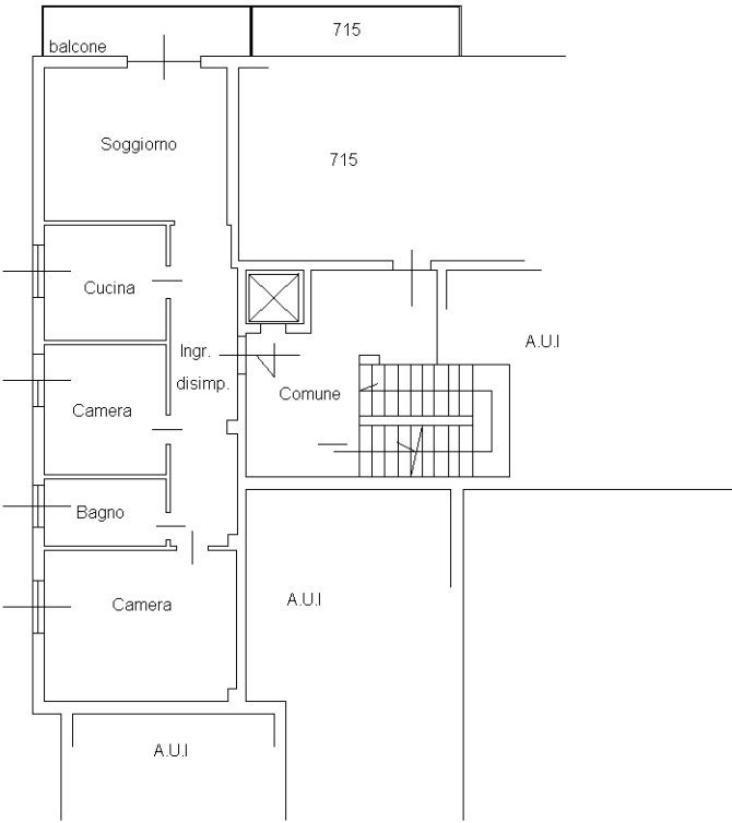
PIANTA SECONDO PIANO H= 3.00
